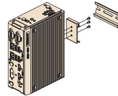
导轨式安装
