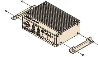
壁挂式安装
